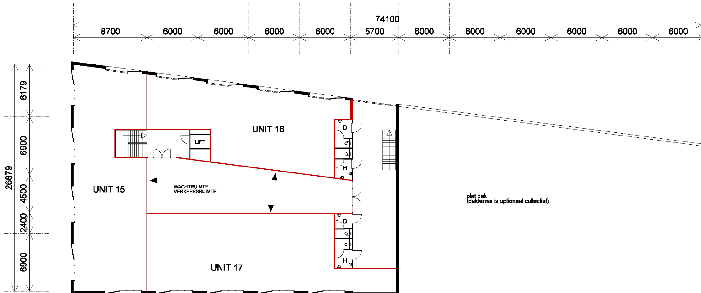
principe plattegrond tweede verdieping
